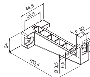
Attacco per finestre a vasistas / Bottom hinged windows bracket
