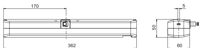
Attuatore Micro + / Micro + actuator
