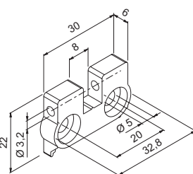
Attacco per finestre a sporgere / Top hinged windows bracket
